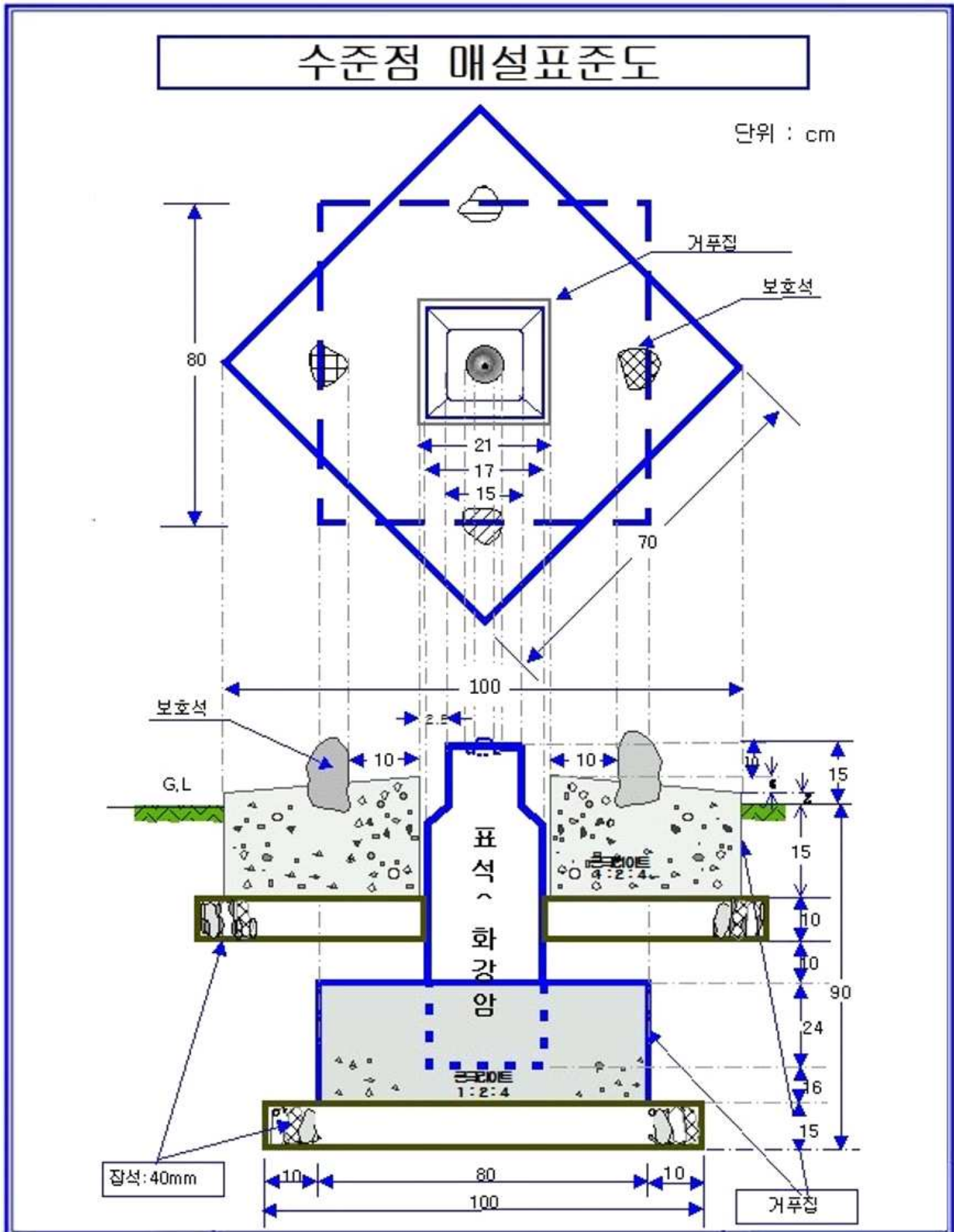
[별표 6-4] 수준점 매설표준도 (제19조제2항 관련)
